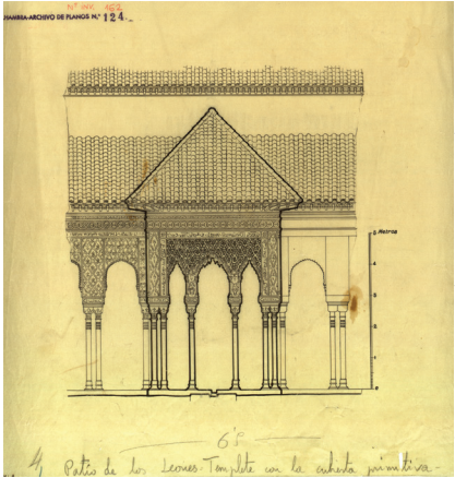
LEOPOLDO TORRES BALBÁS (ARQUITECTO) Y MANUEL LÓPEZ BUENO (DELINEANTE). PATIO DE LOS LEONES. TEMPLETE DE LEVANTE. REPRESENTACIÓN DEL ESTADO ANTERIOR TRAS LA INTERVENCIÓN DE RAFAEL CONTRERAS. 1929 ARCHIVO DE LA ALHAMBRA
