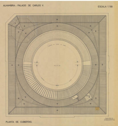
FRANCISCO PRIETO-MORENO PARDO (ARQUITECTO) Y MANUEL LÓPEZ RECHE (DELINEANTE). ALHAMBRA. PALACIO DE CARLOS V. PROYECTO DE LA GALERÍA ALTA. PLANTA DE CUBIERTAS, 1967. ARCHIVO DE LA ALHAMBRA
