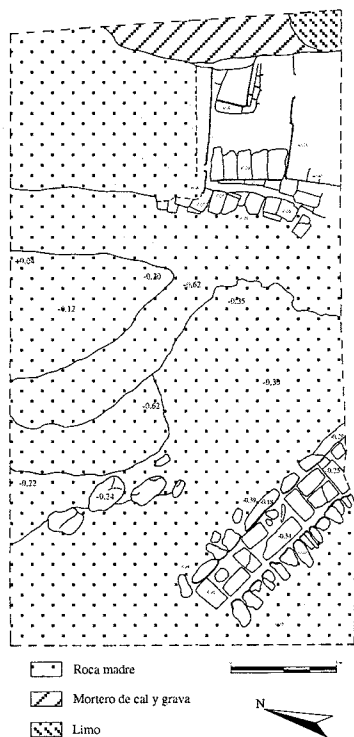
Fig. 4. Planta del sondeo de la galería.
