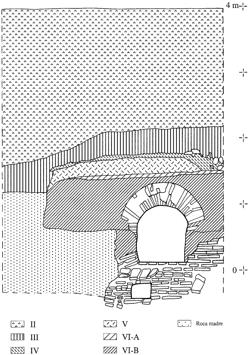
Fig. 5. Perfil E del sondeo de la galería.
