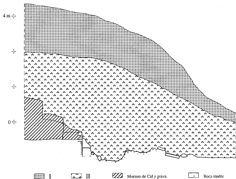
Fig. 7. Perfil S del sondeo de la galería.
