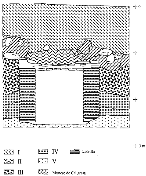
Fig. 3. Perfil E del sondeo del pozo 2.
