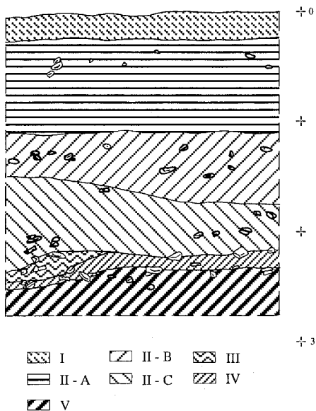
Fig. 2. Perfil S del sondeo del pozo 2.
