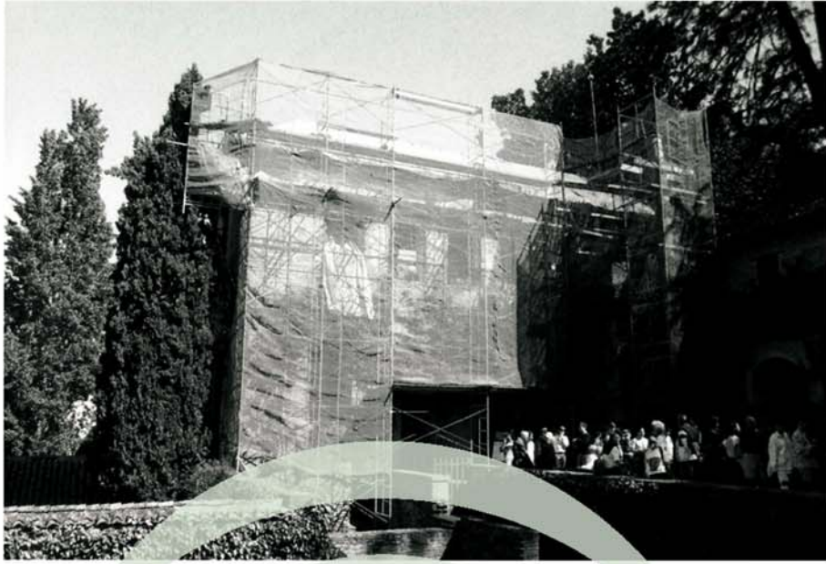
Lám. 10. Trabajos en la cubierta de teja del pabellón sur del Patio de la Acequia.
