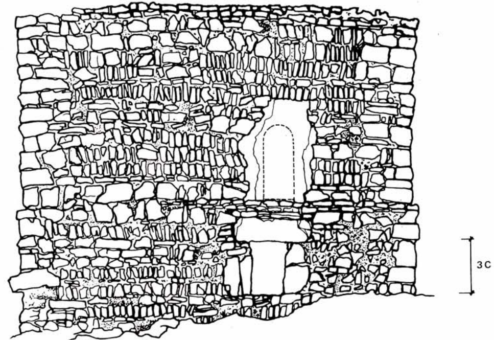
ALZADO SUR
